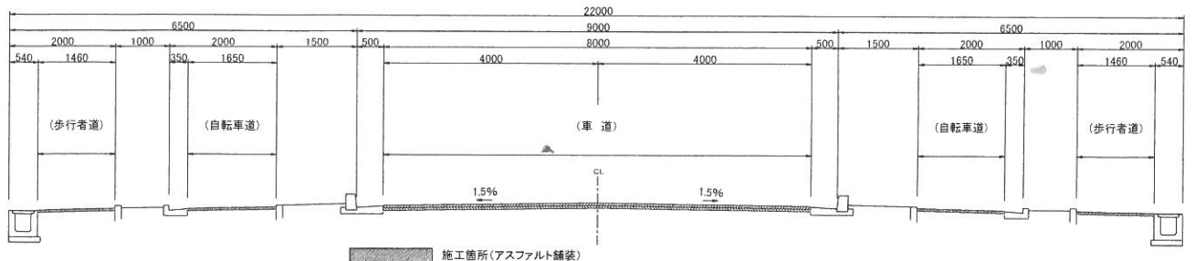
市道0106号線標準横断面図
